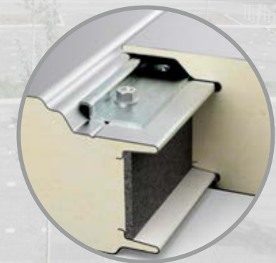
Fuge eines Panels mit verdeckter Befestigung
