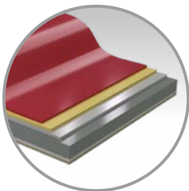
Abb. Exemplarischer Aufbau einer Stahl-Verbundbeschichtung.
