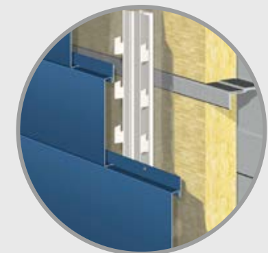
Aufbau VHF mit Kassette und Dämmung
