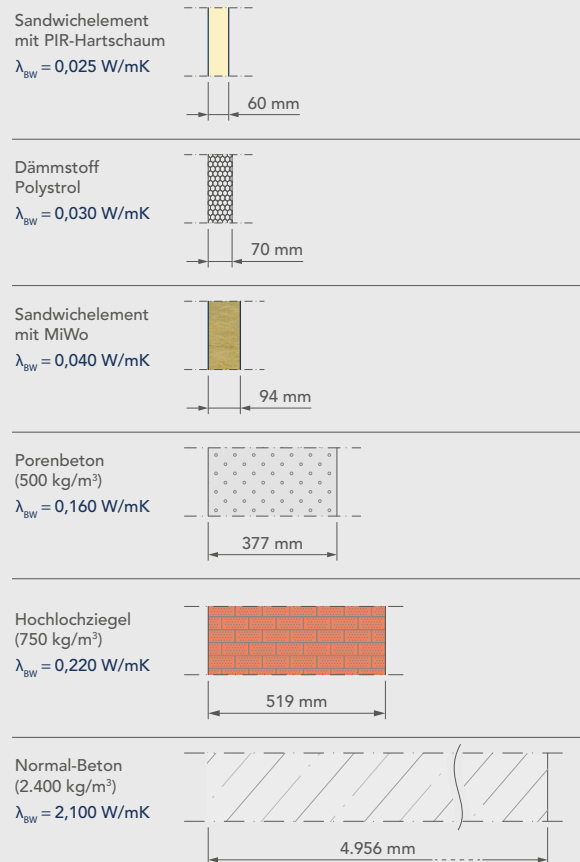
Abb. Unterschiedliche Dämmdicken verschiedener Dämm- und Baustoffe bei gleicher Wärmedämmfähigkeit.
