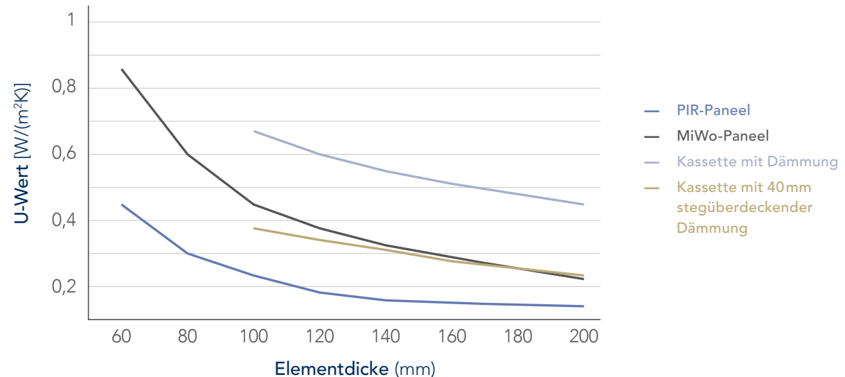
Abb. Wärmedurchgangskoeffizienten in Abhängigkeit der Dämmstärke von Stahl-Sandwichelementen mit Mineralfaser und PIR-Kern im Vergleich zu Kassettenelementen mit Dämmung.
